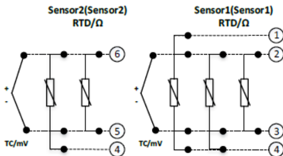
Рисунок 3.4.4 Подключение двух датчиков к преобразователю
