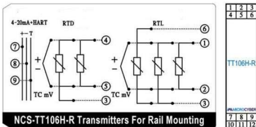
Рисунок 3.7. Подключение датчиков к преобразователю NCS-TT106H-R.
