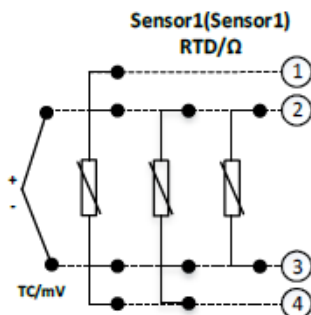
Рисунок 3.4.3 Подключение одного датчика к преобразователю
