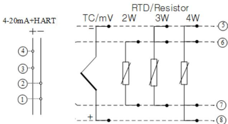
Рисунок 3.6. Подключение датчиков к преобразователю NCS-ТТ106H-R (1).
