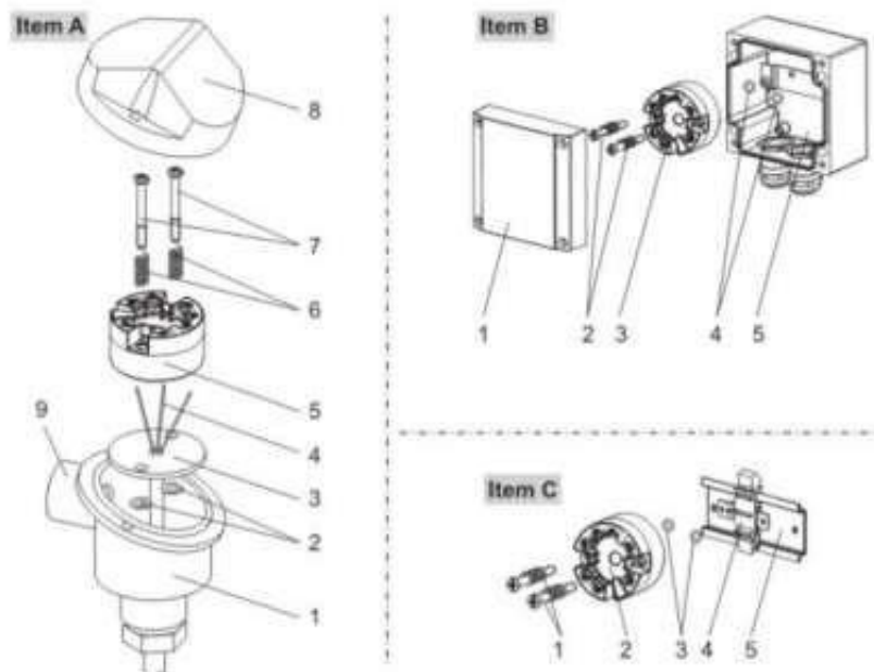
Рисунок 3.2. Установка NCS-ТТ106
