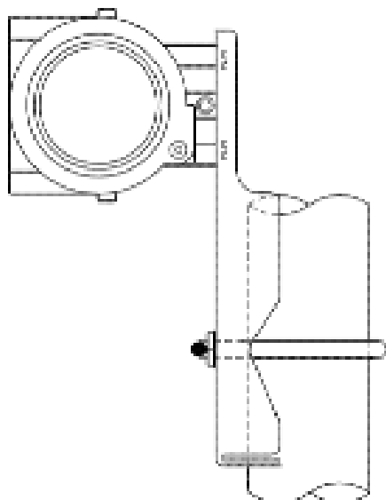
Рисунок 3.1.1 Установка плоского кронштейна для монтажа на трубу
