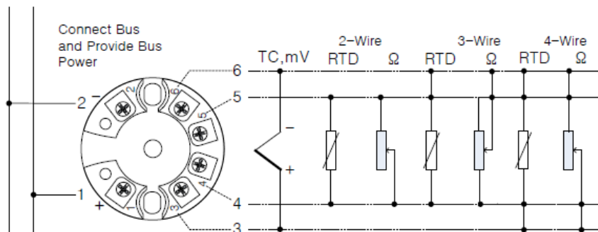
Рисунок 3.5 Подключение датчиков к преобразователю NCS-ТТ106
